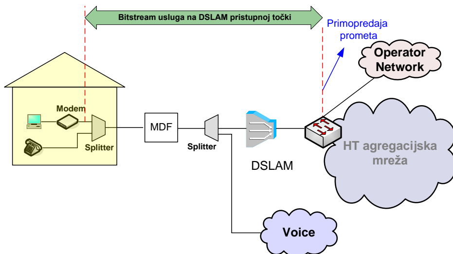
Slika 7. Veleprodajni širokopolasni pristup za pružanje Internet usluge na DSLAM razini u slučaju kada krajnji korisnik ostvaruje Osnovni pristup mreži putem usluge HT-a
